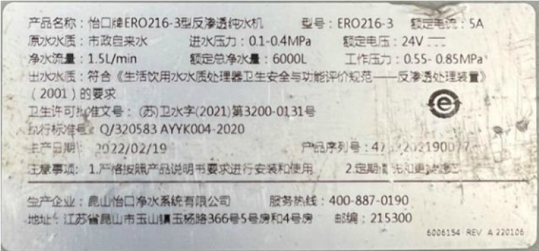
ERO216-3（铭牌）
